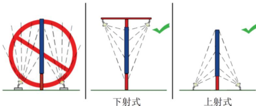
图 5 投射照明方式
