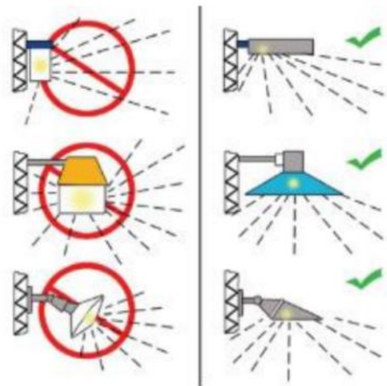
图 4 光源遮蔽方式
